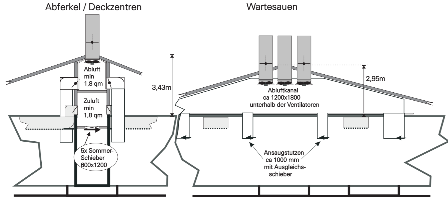
Schnitte vom Lüftungsschema:
